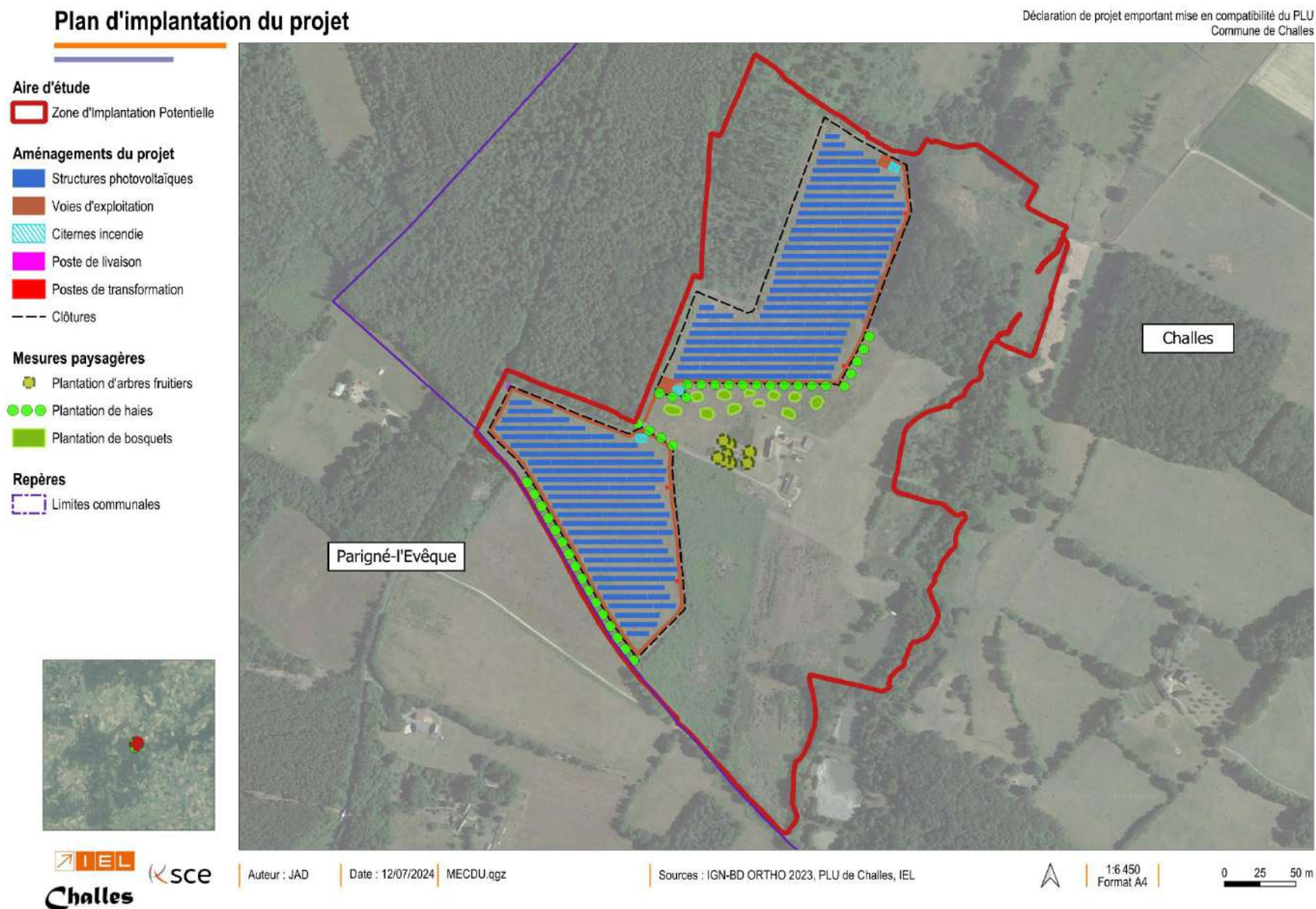
Figure 6 : Plan d'implantation du projet
